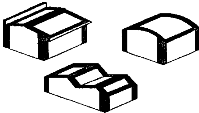
Рисунок 9.11. Ділянки з підвищеним від'ємним тиском вітру
