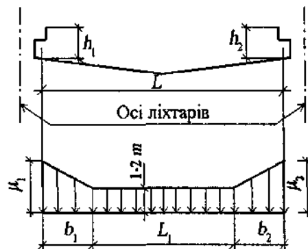
Схема 3'. Будівлі з поздовжніми ліхтарями, відкритими зверху
