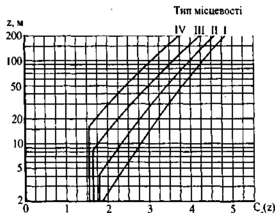
Рисунок 9.2. Коефіцієнт висоти споруди C_h .
