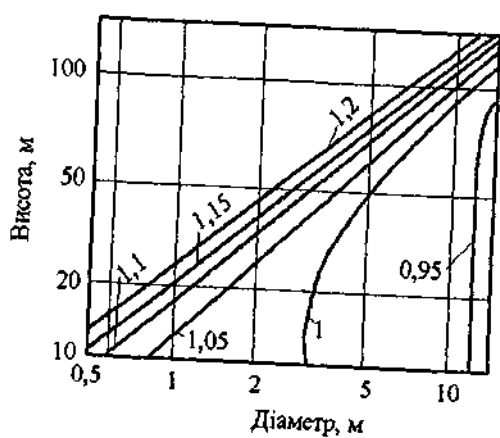
Рисунок 9.8. Коефіцієнт C_d для сталевих труб і апаратів колонного типу без футерівки
