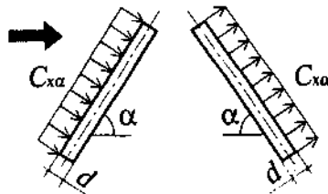
Схема 19. Ванти та нахилені трубчасті елементи, розташовані у площині потоку
