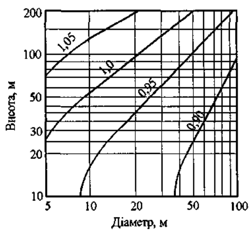
Рисунок 9.7. Коефіцієнт C_d для будівель із сталобетонним каркасом
