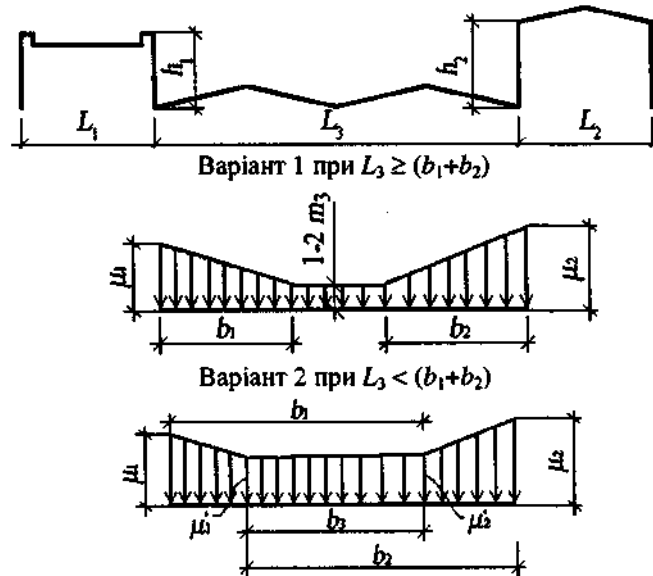
Схема 9. Будівлі з двома перепадами висоти
