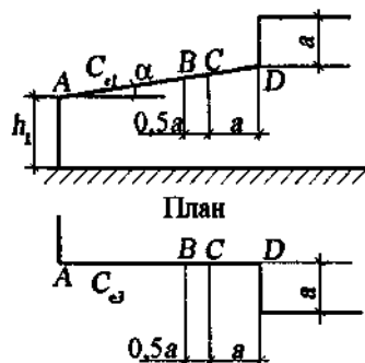
Схема 10. Уступи будівель при \alpha < 15^\circ
