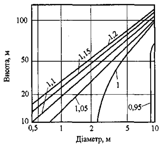
Рисунок 9.9. Коефіцієнт C_d для сталевих труб і апаратів колонного типу з футерівкою
