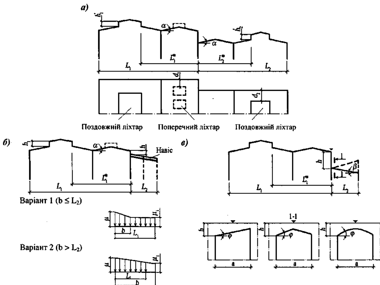
Схема 8. Будівлі з перепадом висоти
