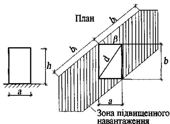
Схема 11. Ділянки покриттів, що примикають до вентиляційних шахт, які вивисуються над покрівлю, та інші надбудови
