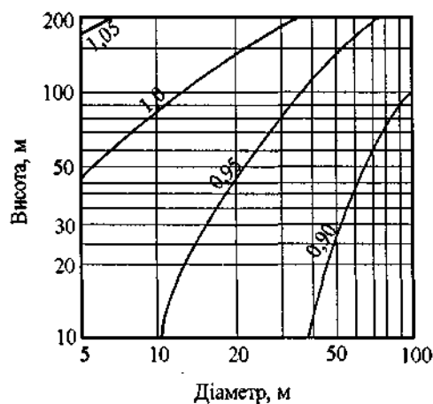
Рисунок 9.5. Коефіцієнт Q для кам'яних будівель і будівель із залізобетонним каркасом
