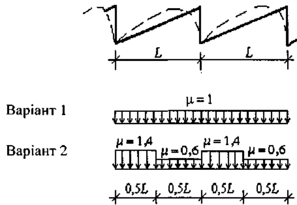
Схема 4. Шедові покриття
