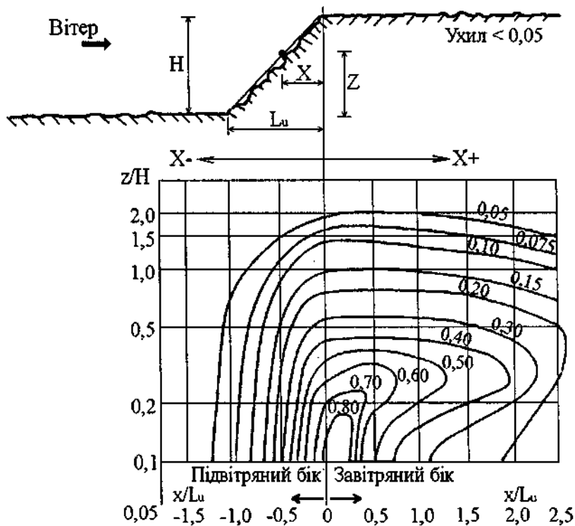
Рисунок 9.3. Коефіцієнт S для схилів
