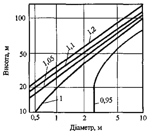
Рисунок 9.10. Коефіцієнт C_d для залізобетонних труб
