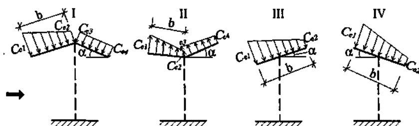
Схема 11. Навіси
