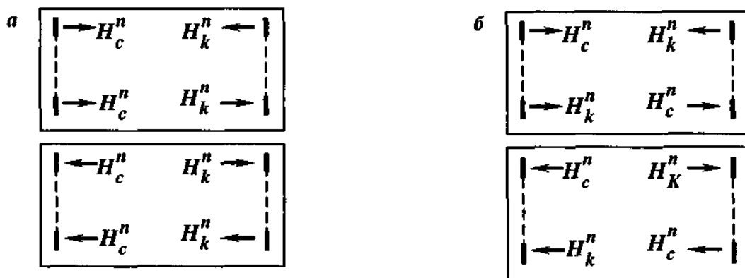
Рисунок 7.1. Варіанти прикладення бічних сил для чотириколісних кранів
