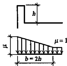
Схема 10. Покриття з парапетами
