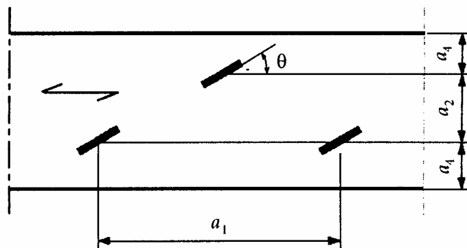
Рисунок 13.10 – Визначення кроку скоб
