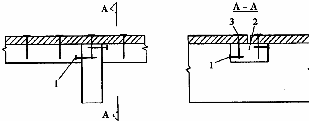
Рисунок 15.1 – Приклад кріплення панелей, що не обпираються на балки або крокви
