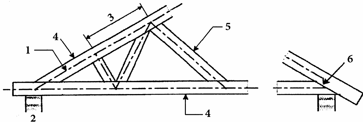
1 – лінія розрахункової моделі; 2 – опора; 3 – проліт; 4 – зовнішній елемент; 5 – внутрішній елемент; 6 – фіктивний балочний елемент
