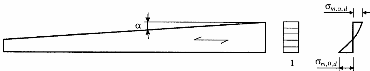
Рисунок 11.8 – Односкатна балка
