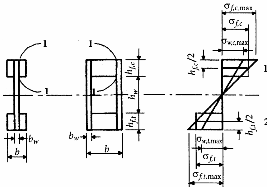
Рисунок 14.1 – Тонкостінні балки
