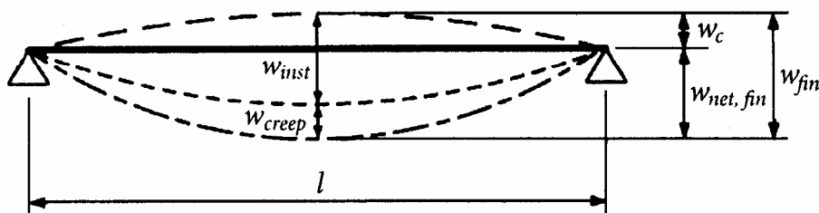
Рисунок 12.1 – Складові прогину
