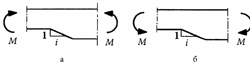
Рисунок 11.10 – Згин у підрізці
