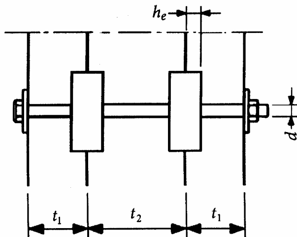
Рисунок 13.12 – Розміри з'єднання з розрізними і гладкими кільцевими шпонками
