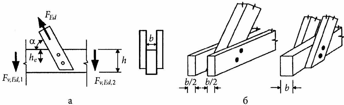
Рисунок 13.1 – Передача з'єднанням зусиль під кутом
