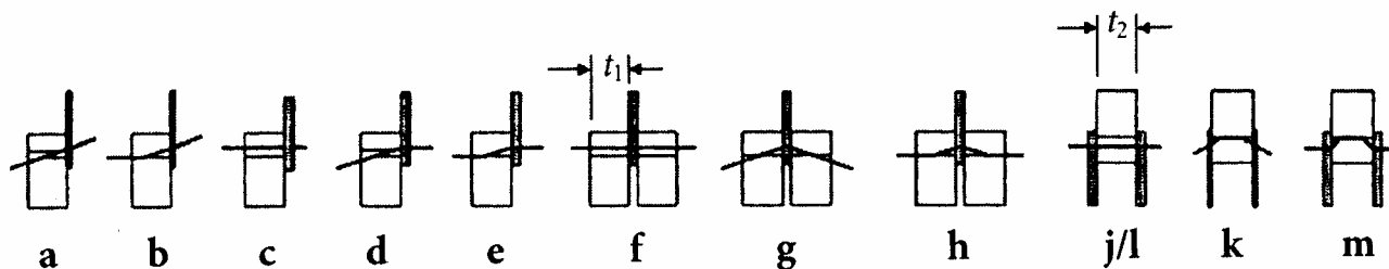
Рисунок 13.3 – Моделі руйнування для з'єднань "сталь-брус"
